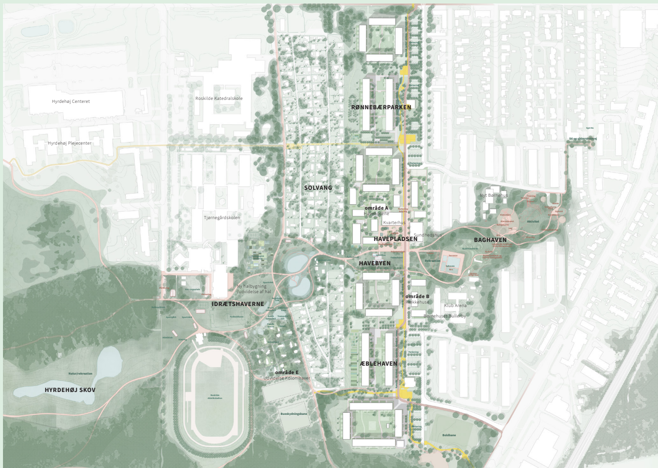
Situationsplan vinderforslag
